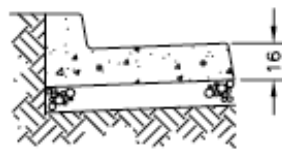
尺寸界线外部的文字与尺寸线对齐
